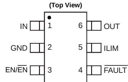
SOT26
